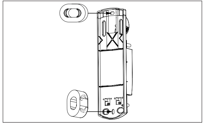
Abb. 2 Einclipsen der separaten Abstandhalter ins Schraubloch
