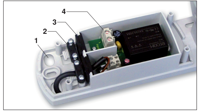
Abb. 7 Anschluss der Wetterstation
